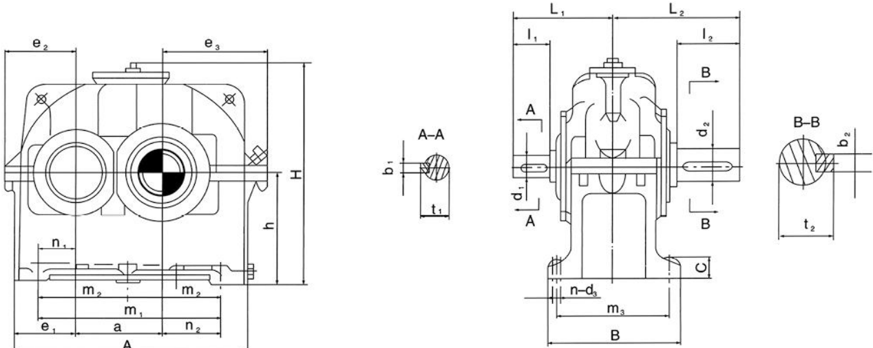
YFZDY YFZDZ型装配型式 YFZDY YFZDZ Design
