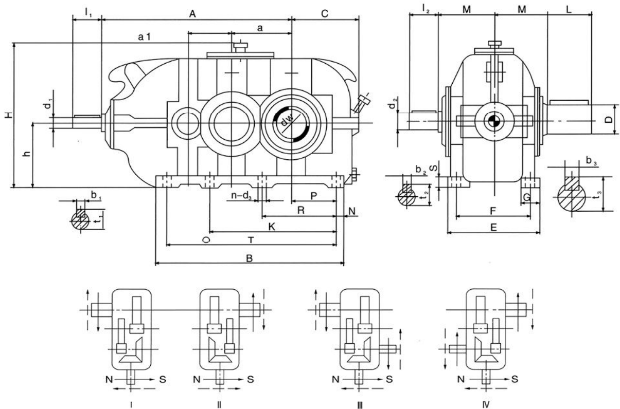
YFDCY、YFDCZ型装配型式 YFDCY、YFDCZ Design 图7
