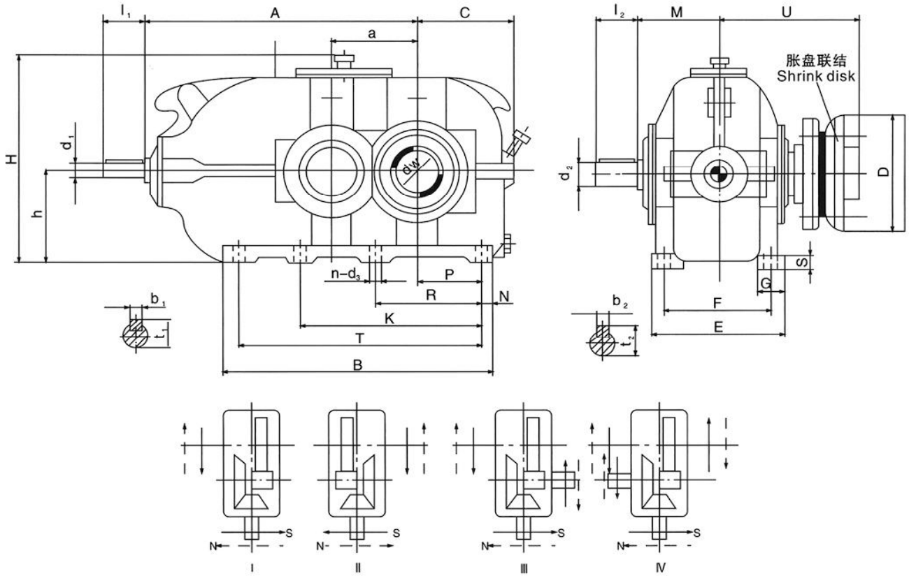
YFDBYK型装配型式 YFDBYK Design 图6
