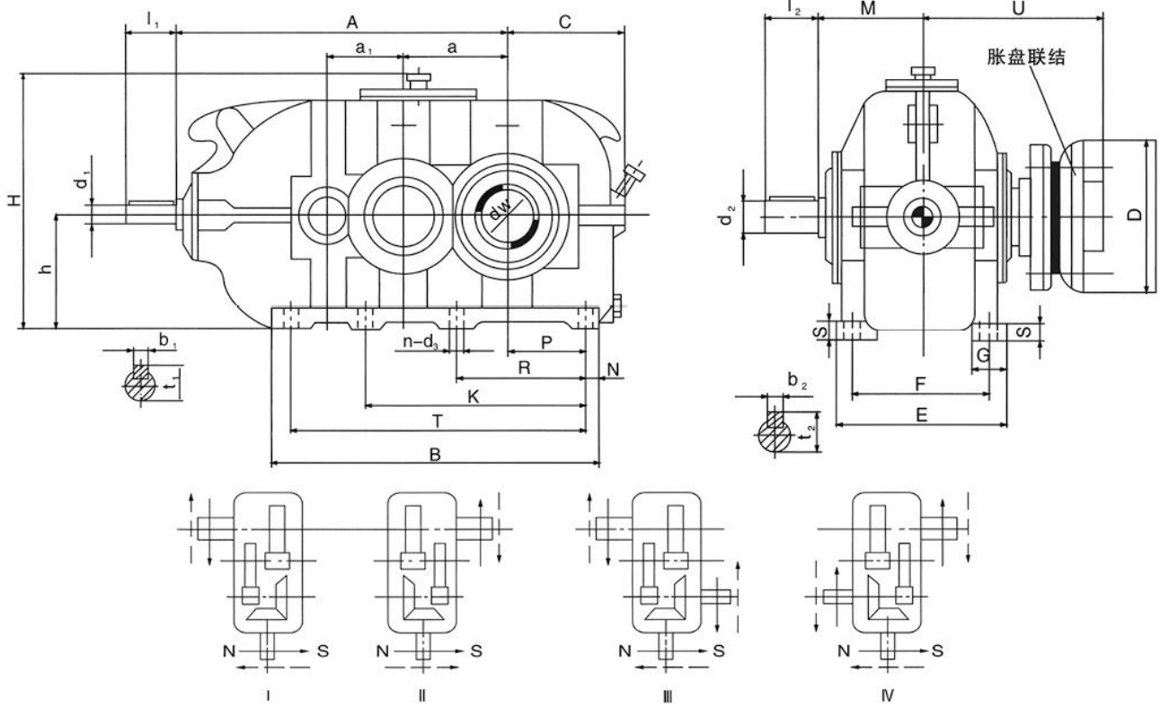
YFDCYK型装配型式 YFDCYK Design
